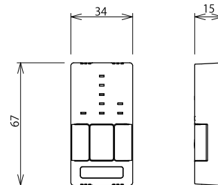
リモコン外形図 (Free)
